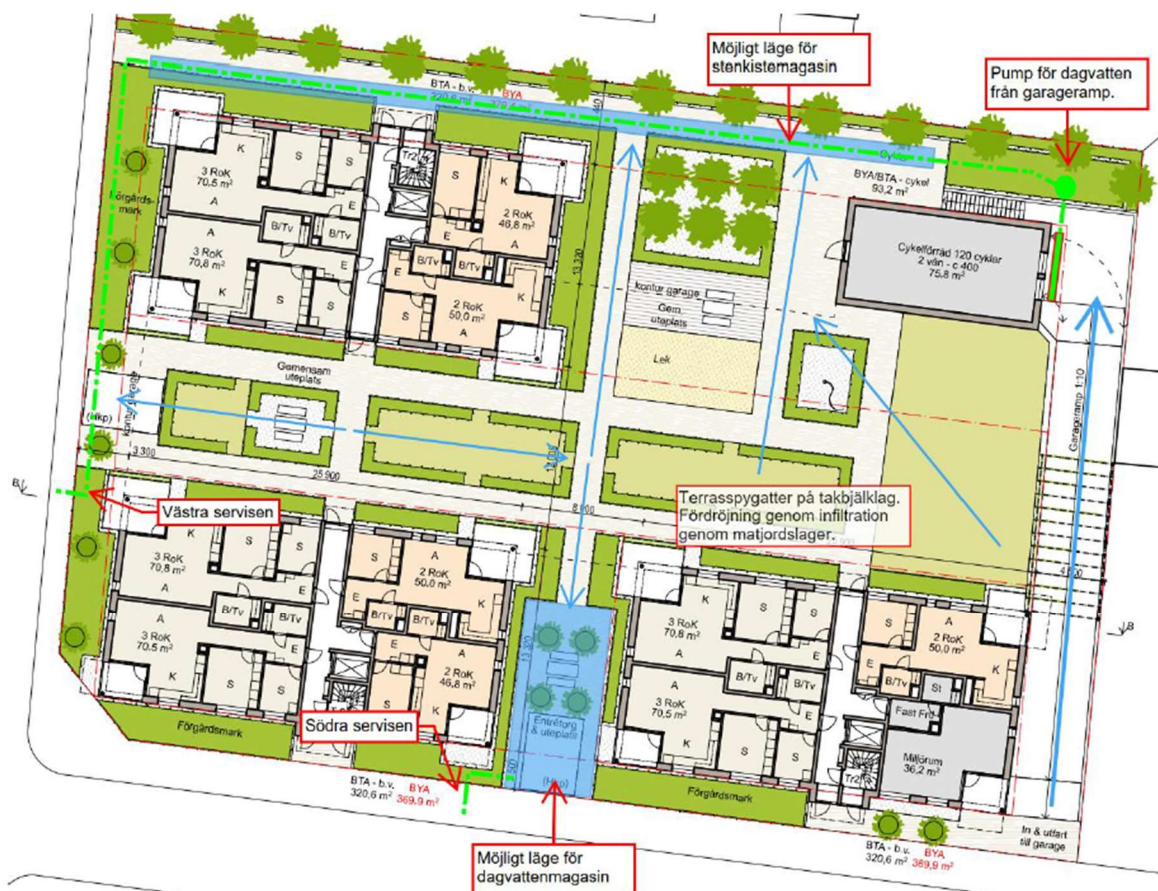
Exempel på principlösning för dagvatten inom fastigheten. Utdrag ur dagvattenutredning.
