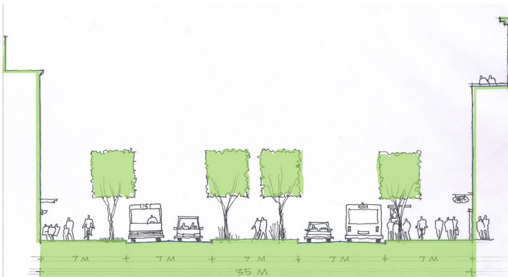
Gatusektion Teleborgsvägen.
